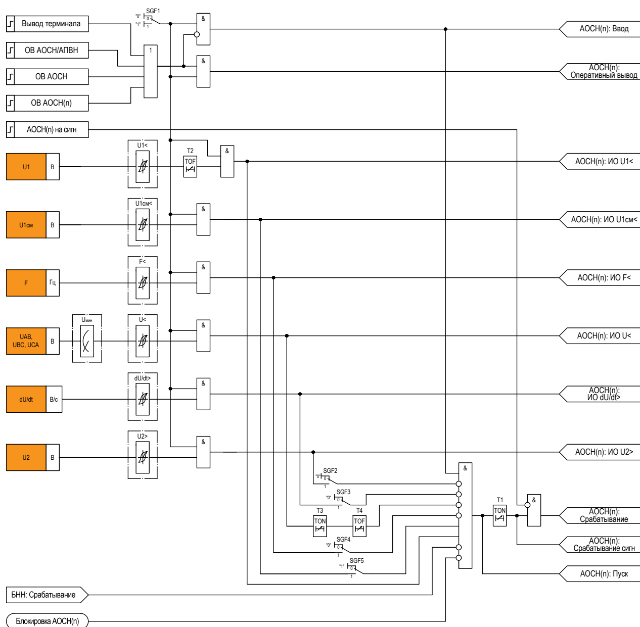
Рисунок 2.5 – Функциональная схема логики очереди АОСН
